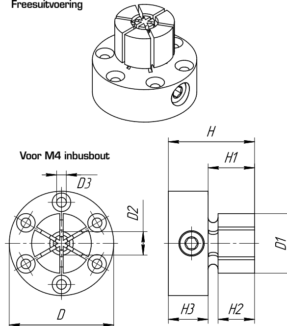
Freesuitvoering
