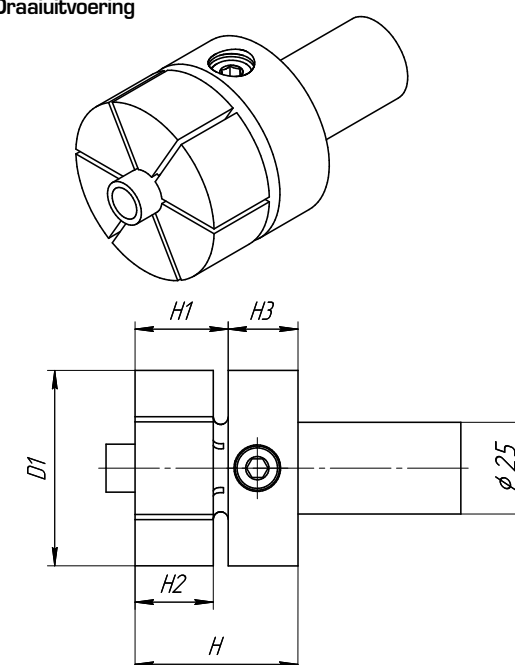
Draaiuitvoering
